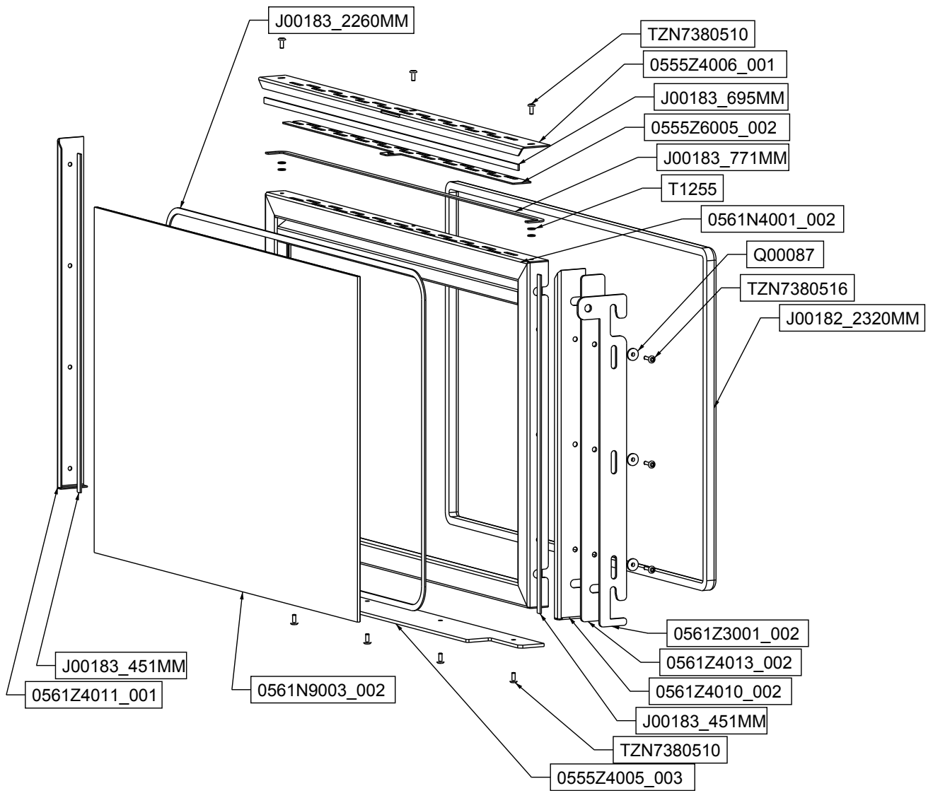
FIG.1-B - STILKAMIN S-460
