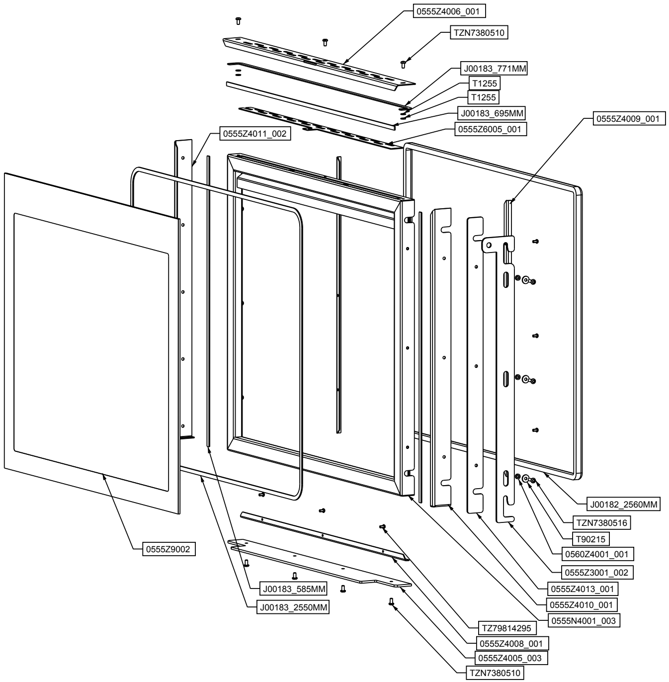
FIG.1-A - STILKAMIN S-600
