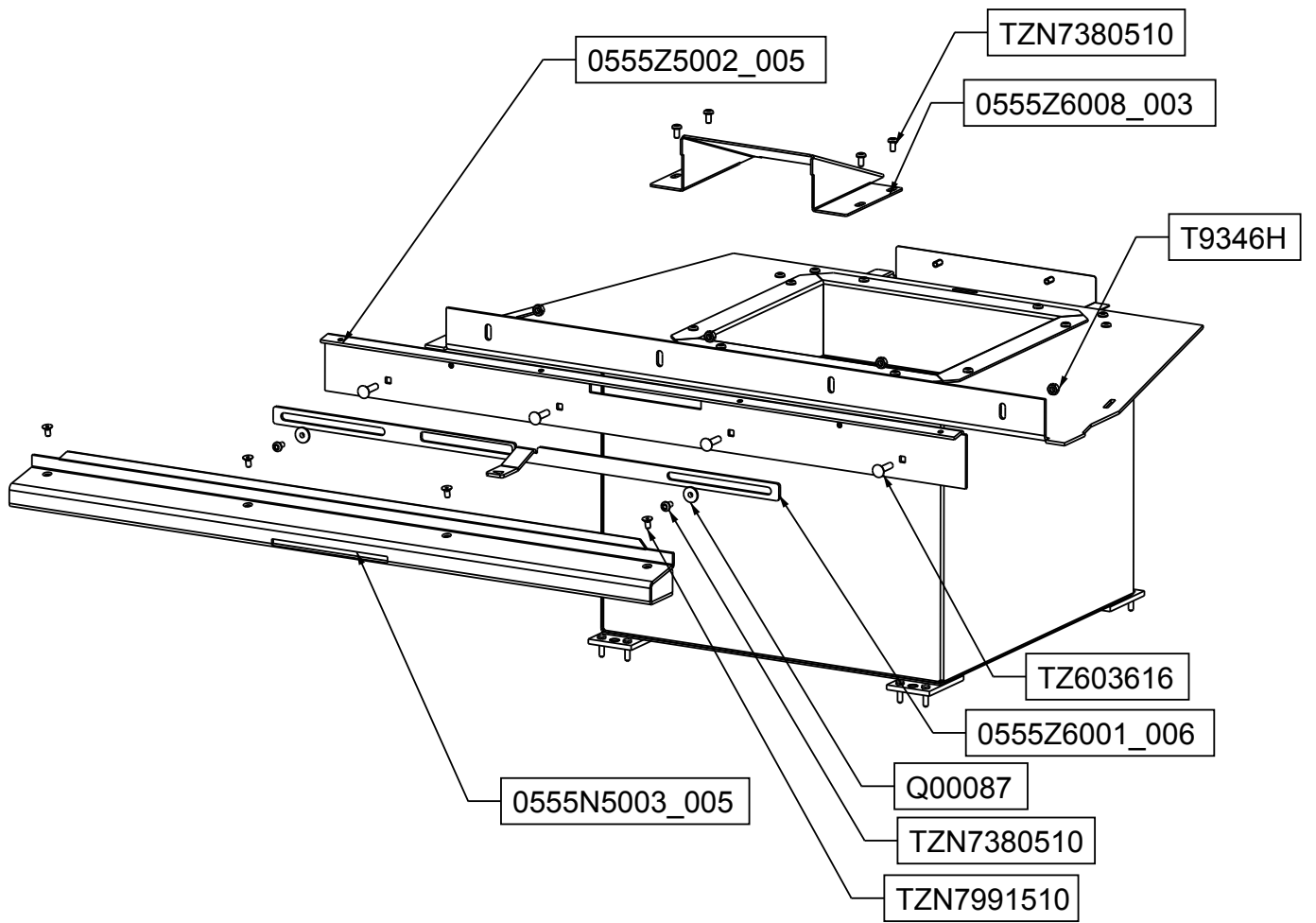
FIG.2 - STILKAMIN S-600/STILKAMIN S-460
